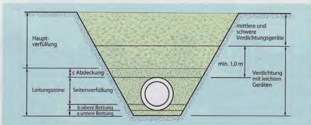
Zulässige Verdichtungsgeräte.
