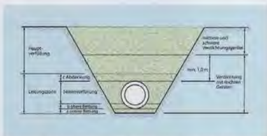
Zulässige Verdichtungsgeräte
