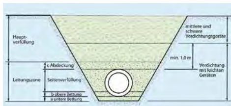
Zulässige Verdichtungsgeräte
